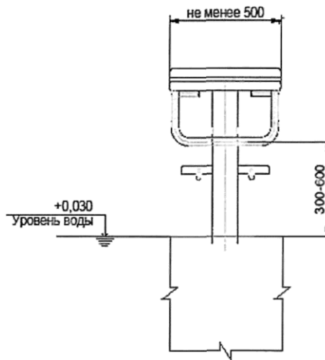
Рис. 5.3 - Устройства и размеры стартовых тумбочек
